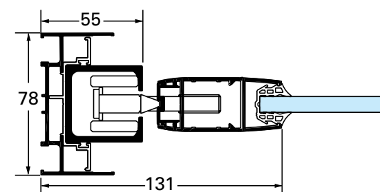
Full-access door
